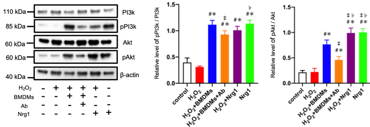
図3. Neuregulin 1-ErbB-PI3K-Akt シグナル伝達経路の活性制御機構
